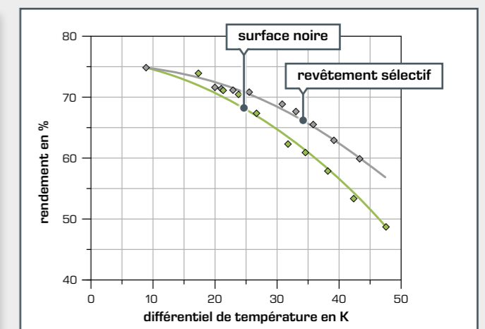
L'efficacité dépend de la température du capteur. Un revêtement spécial de l'absorbeur permet d'obtenir des rendements plus élevés.
