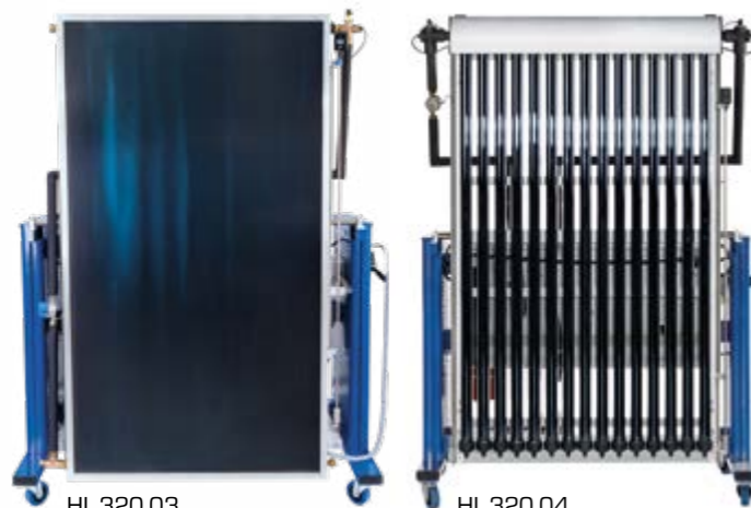
HL 320.03 Capteur plan
