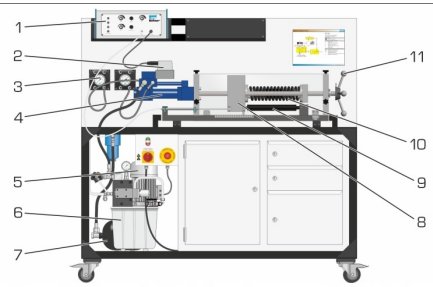
1 amplificateur de régulation, 2 soupape de régulation, 3 manomètre de pression de cylindre, 4 vérin hydraulique, 5 pompe, 6 réservoir d'huile, 7 accumulateur hydraulique, 8 chariot, 9 amortisseur, 10 ressorts, 11 molette de réglage du ressort
